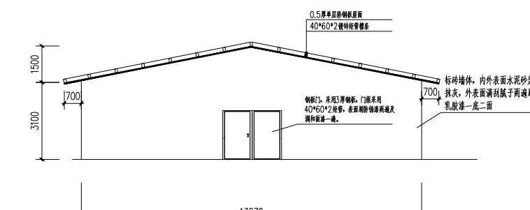
库房正立面图
