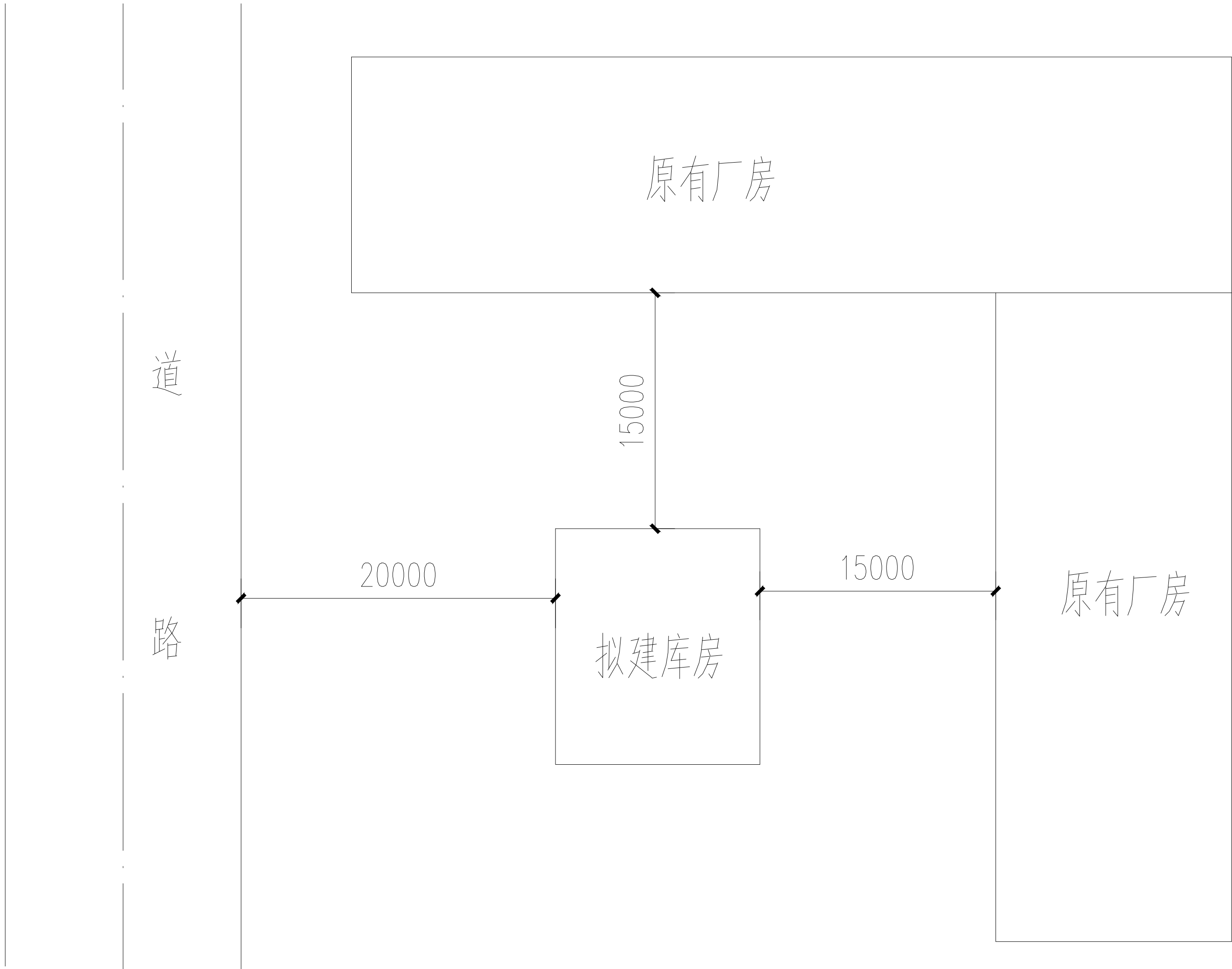
库房总平面图
