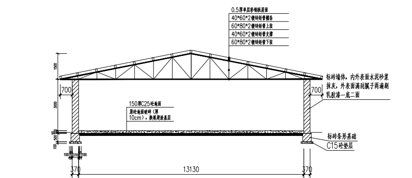
库房剖面图
