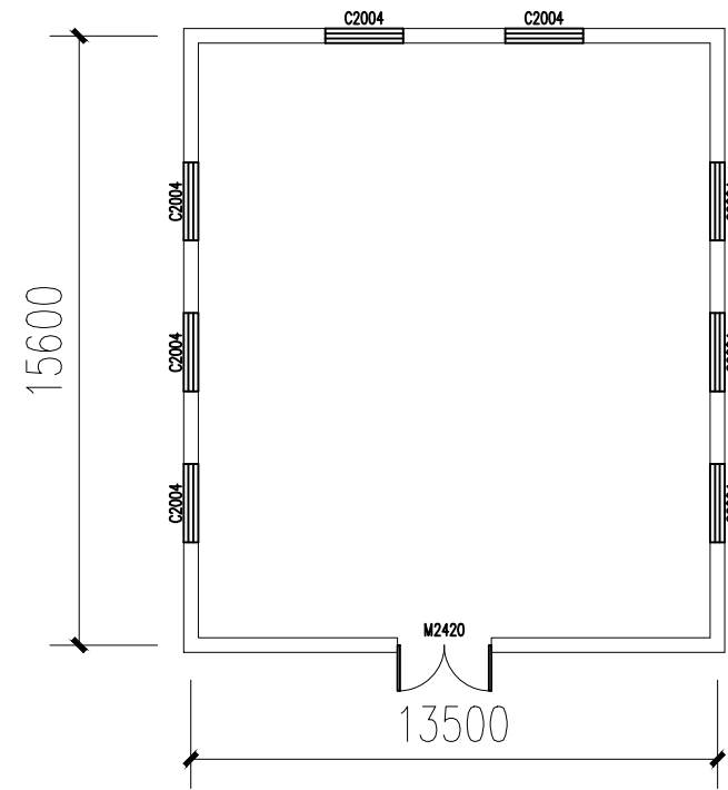
库房平面图
