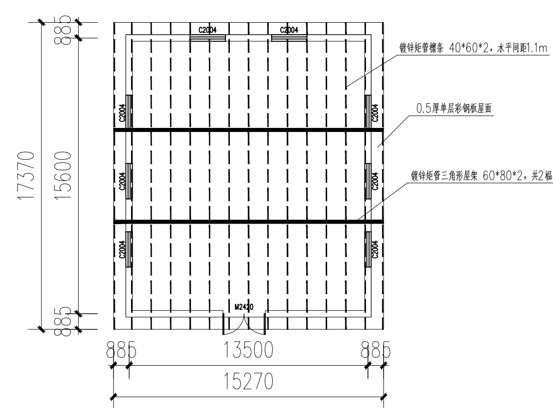
库房屋面钢结构平面图
