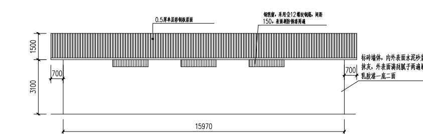
库房侧立面图
